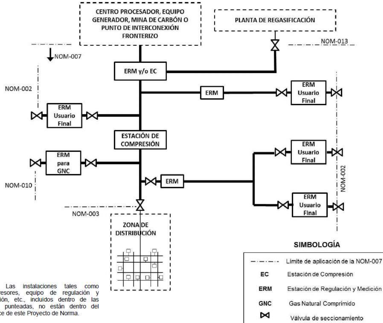
Diagrama 1: Instalaciones de un sistema de transporte que están dentro del alcance de este Proyecto de Norma.
