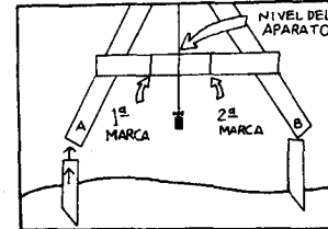
8. El sitio entre las dos marcas es el nivel del aparato. Nivela las estacas hasta que coincidan con el hilo de la plomada, invierta la posición y verifique.
