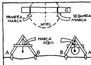
7. Marque en "C" el lugar por donde pasa el hilo de la plomada, invierta la posición del aparato y vuelva a marcar en "C".
