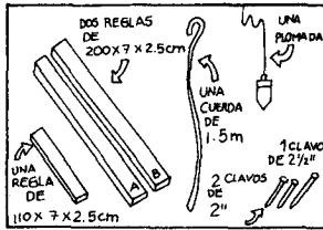
1. Reunir el material.
