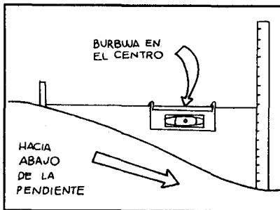
3. Poner la cuerda a nivel. Medir en el extremo cuántos centímetros de altura de diferencia tiene en estos dos metros.
