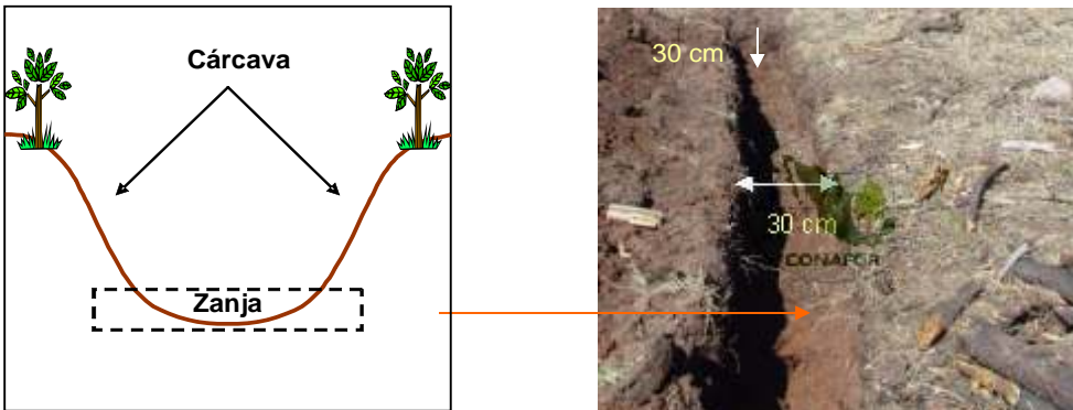
Figura 44. Sección transversal de una cárcava y área de corte para zanja
