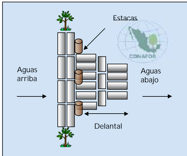
Figura 69 Diseño de presa de costales con delantal
