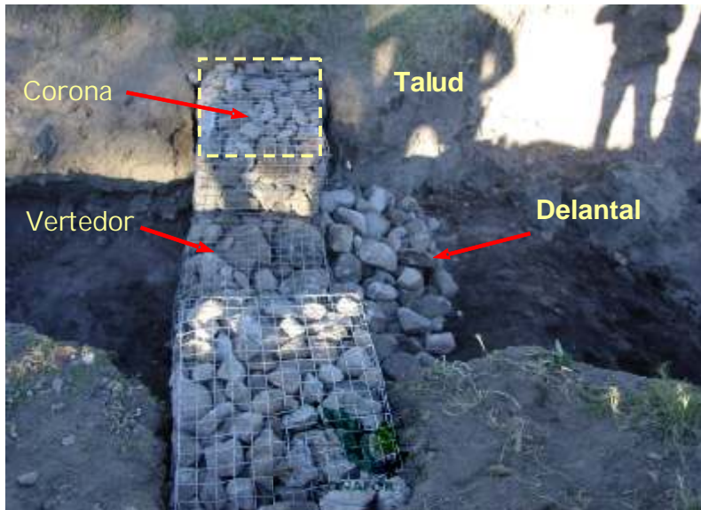
Figura 25. Vertedor en una presa de malla
