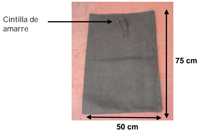
Figura 72. Dimensiones de geocostales utilizados en presas para control de azolves
