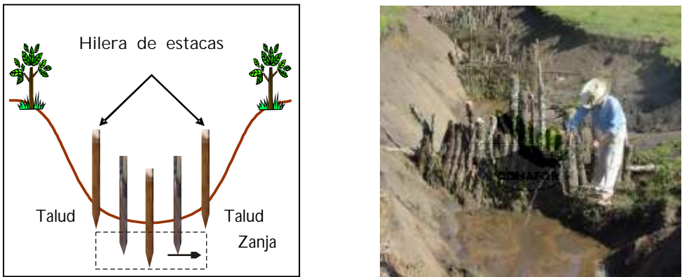
Figura 45. Colocación transversal de hilera de estacas
